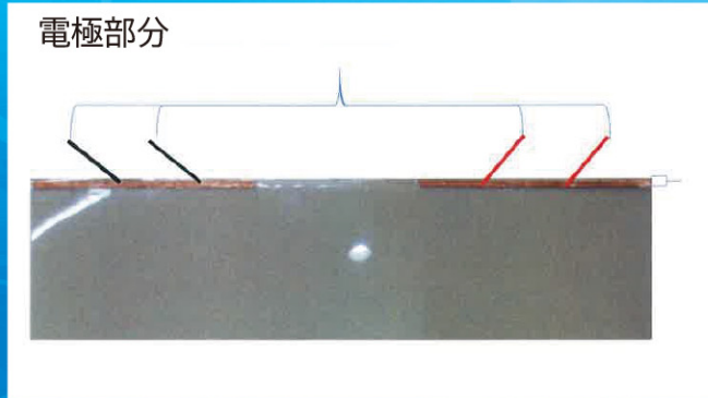
一枚のフィルムに対して、左右2箇所 に電極が取り付けられておりそれぞれの電極に配線が2本ずつ 結線されている
